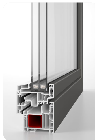
NOVO SE Design 100% renforcée avec ouvrant-dormant affleurants à l'extérieur pour encore plus de modernité.
