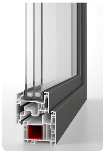
NOVO SE 100% renforcée en acier et Powerdur® hybride pour encore plus de performance thermique.
