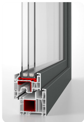
NOVO S 100% renforcée en acier ouvrant et dormant pour plus de sécurité.
