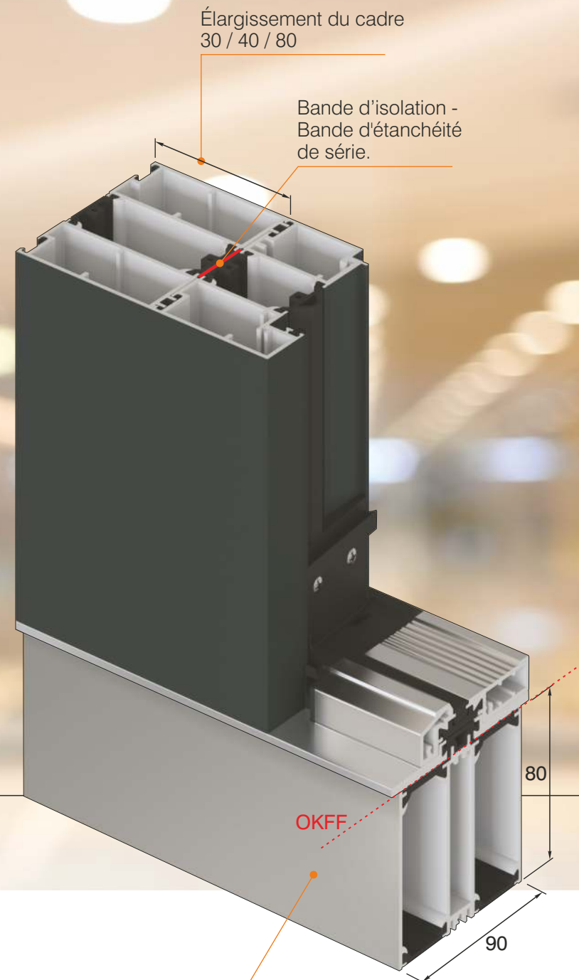
Profil d'encastrement au sol 30 / 40 / 80 mm
