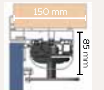
Coupe précadre et capot
